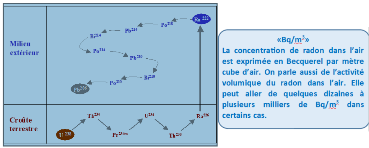
Figure 2 : Chaîne de désintégration de l'Uranium 238 et du Radon 222
