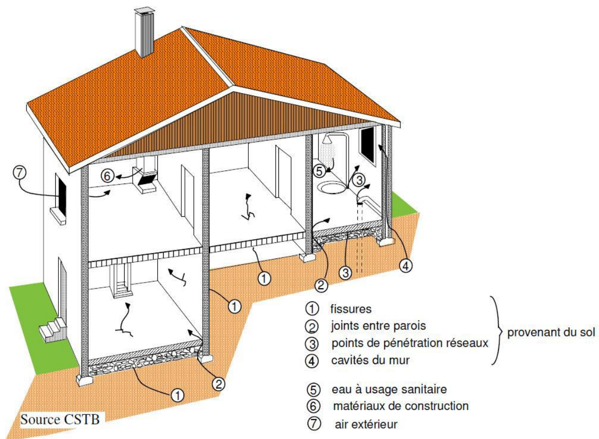
Figure 5 : Voies d'entrée du radon dans les bâtiments
