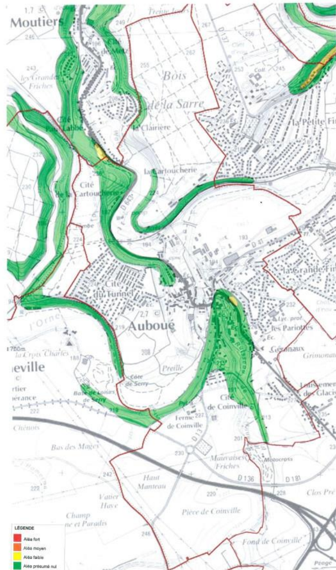
CARTE ALEA CHUTES DE BLOCS BRGM Septembre 2008
