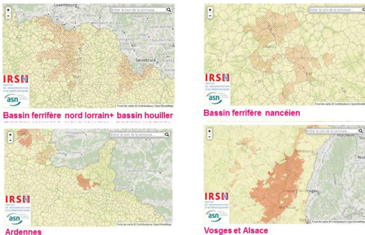
Figure 6 : Zone à risque Radon (source IRSN/ASN)
